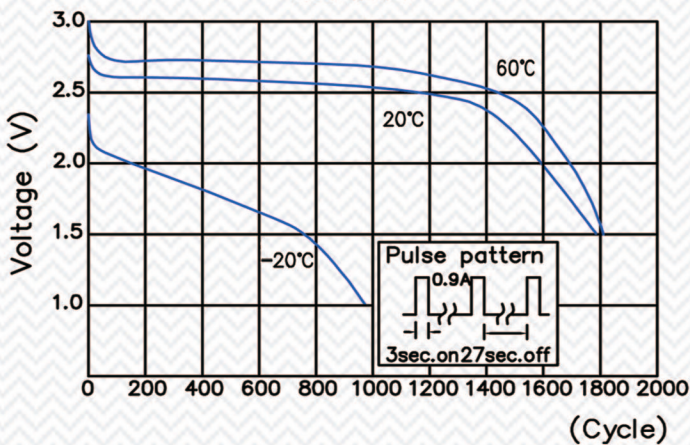
脉冲放电图
