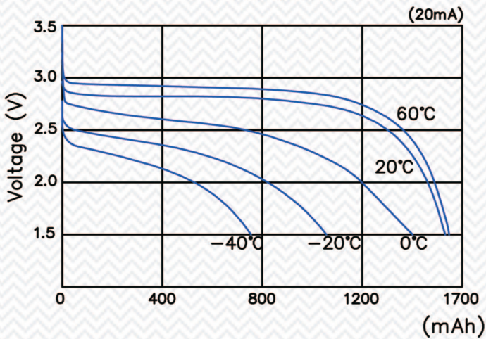
20mA 放电曲线图
