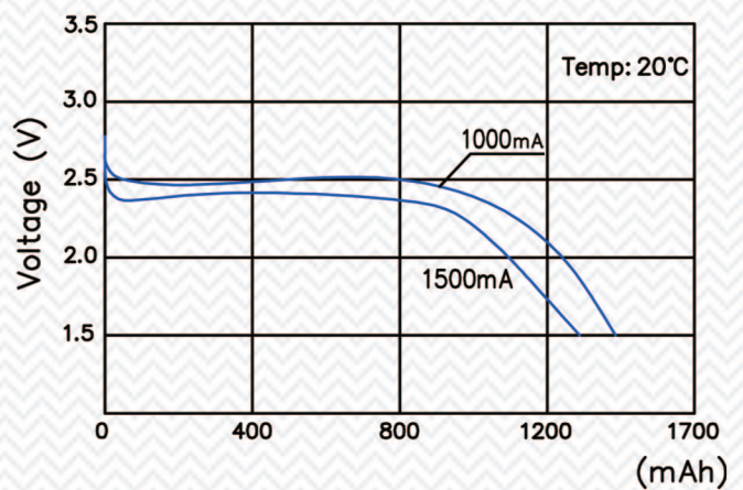
大电流放电图
