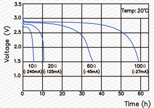
大电流放电图
