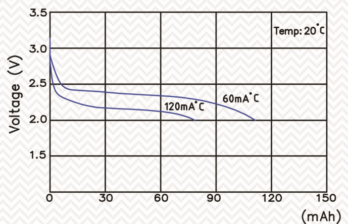
大电流放电图
