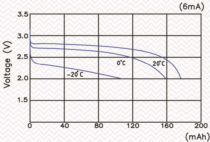
6mA 放电曲线图
