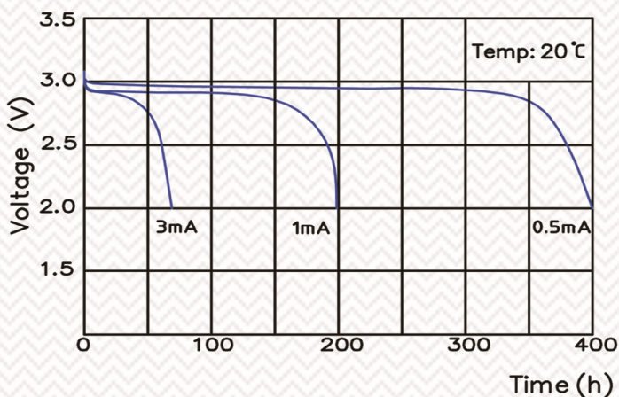
脉冲放电图
