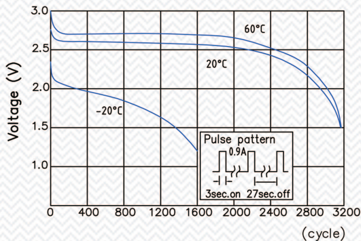
脉冲放电图
