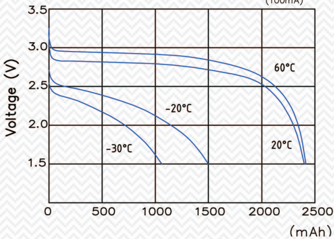
100mA 放电曲线图 (100mA)
