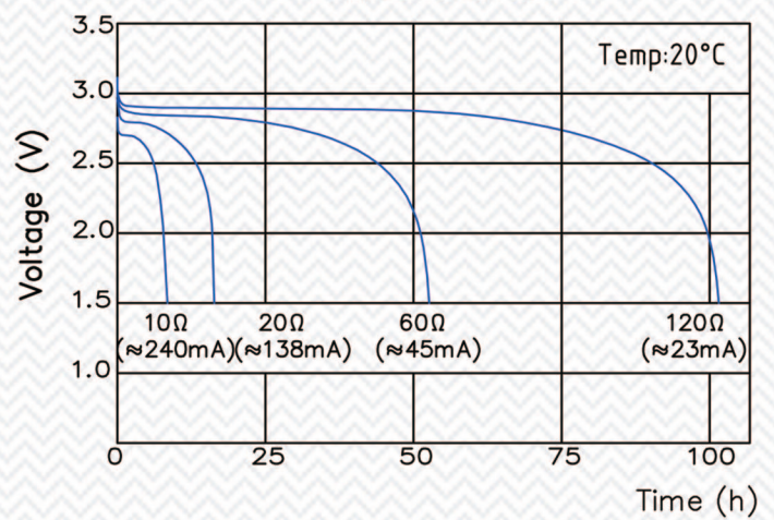
不同电阻放电曲线图
