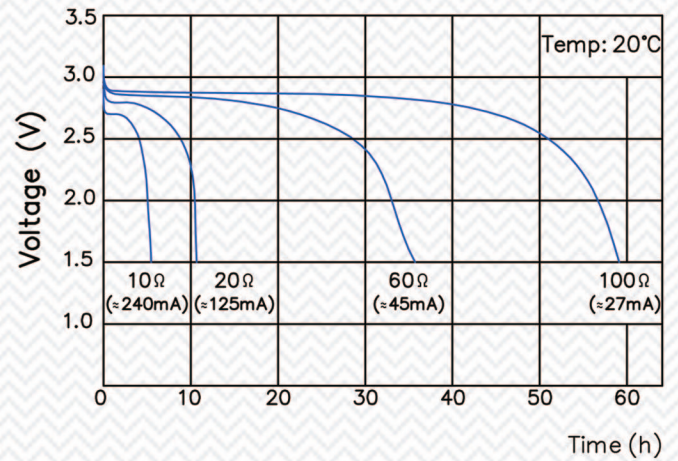
不同电阻放电曲线图
