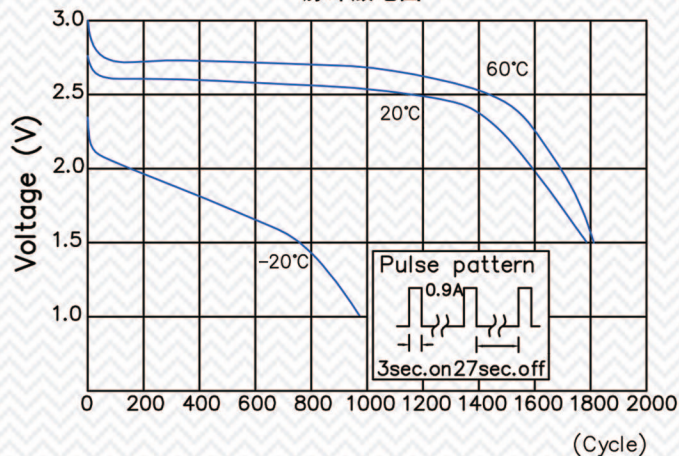
脉冲放电图
