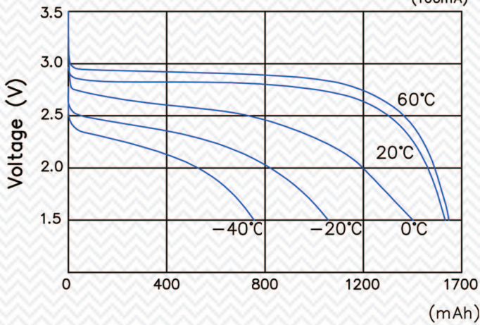
100mA 放电曲线图
