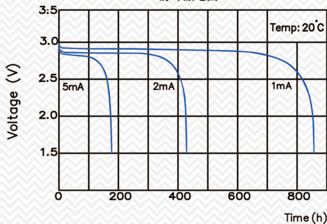
脉冲放电图
