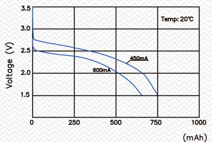
大电流放电图
