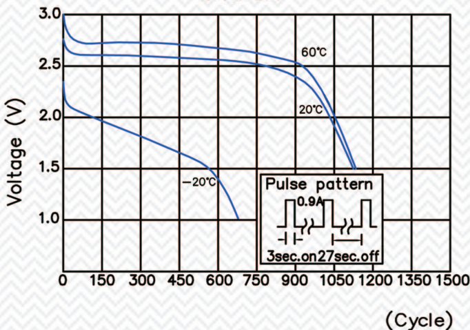
脉冲放电图
