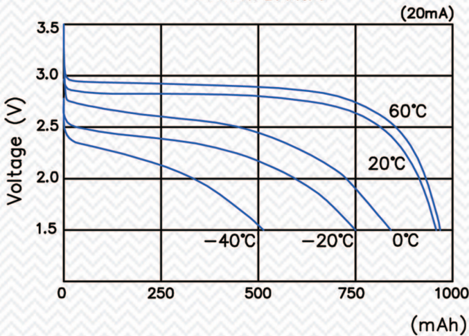
20mA 放电曲线图
