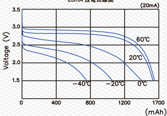
20mA 放電曲線圖
