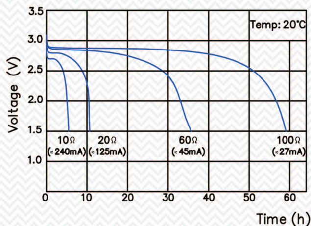
不同電阻放電曲線圖
