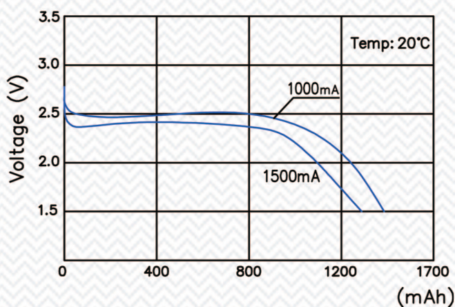
大電流放電圖
