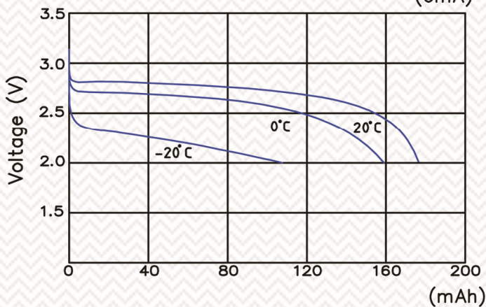
6mA 放電曲線圖 (6mA)
