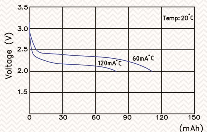
大電流放電圖
