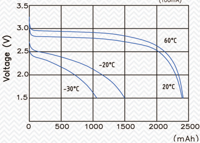
100mA 放電曲線圖 (100mA)
