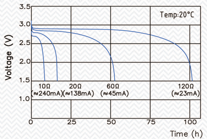
不同電阻放電曲線圖
