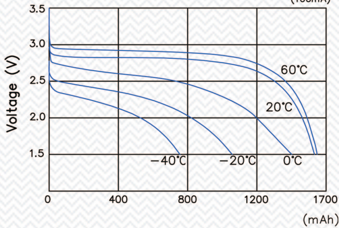
100mA 放電曲線圖
