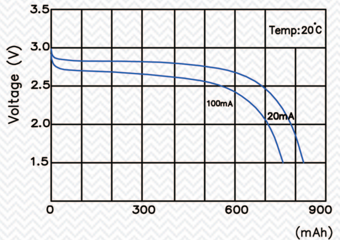
不同電阻放電曲線圖
