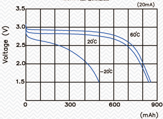
20mA 放電曲線圖
