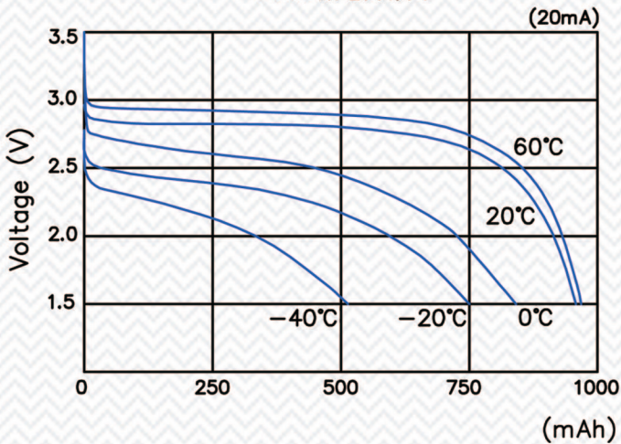
20mA 放電曲線圖
