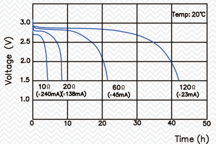
大電流放電圖
